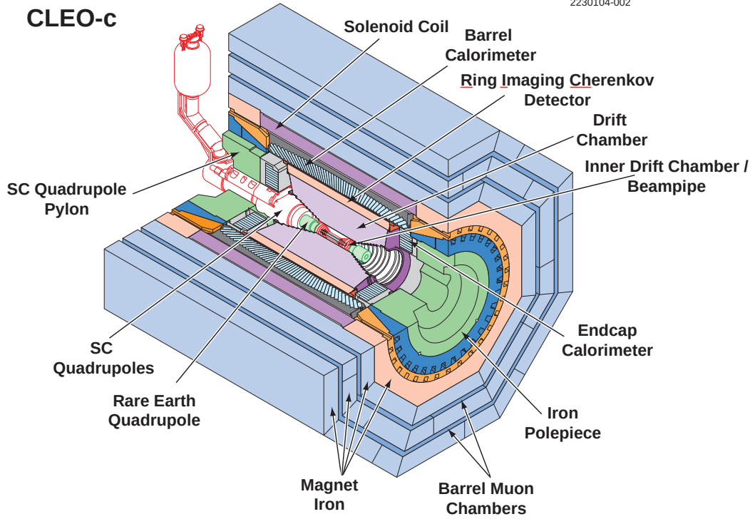
Fig. 2.2: CLEO-c.
